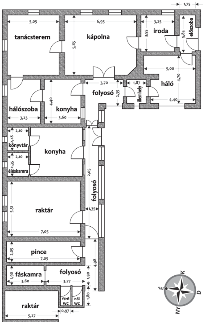
A tótteleki parókia alaprajza
