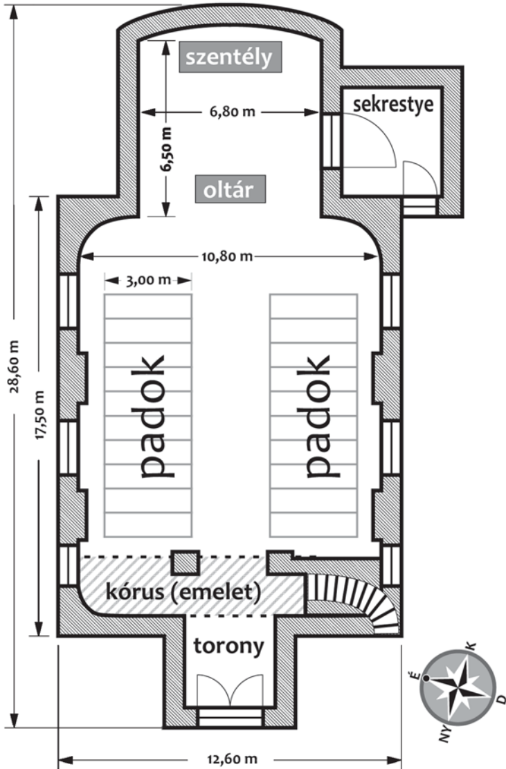
A tóttelkei római katolikus templom alaprajza
