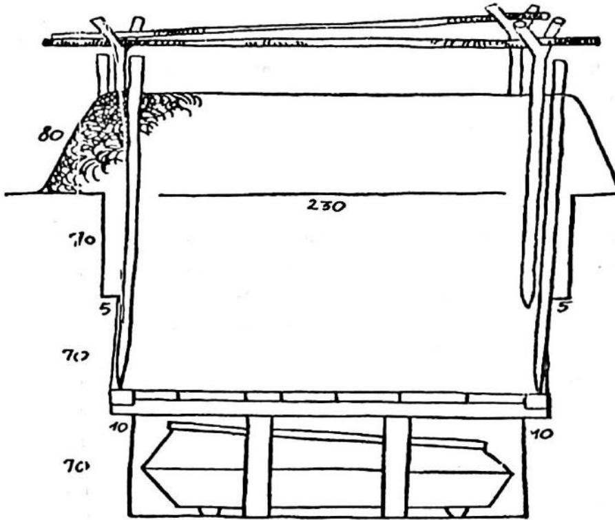
Padmolyos sír oldalmetszete
