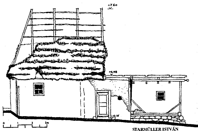
Zsúpfedeles ház – udvar felőli homlokzat
