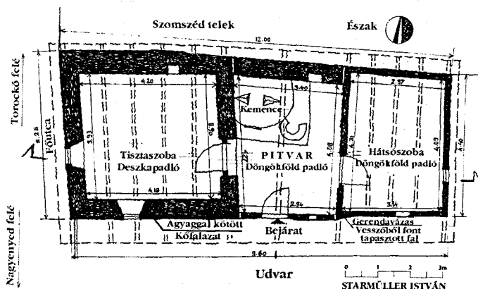
Zsupfedeles ház – alaprajz
