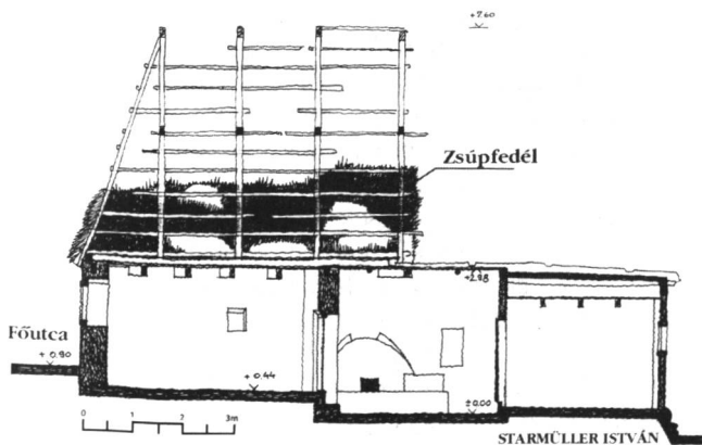
Zsúpfedezés ház – hosszmetesz
